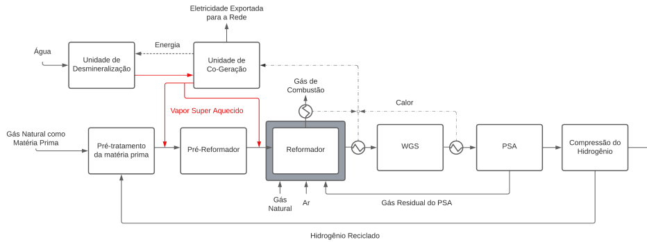
Figura 2. Esquema de uma planta SMR.
