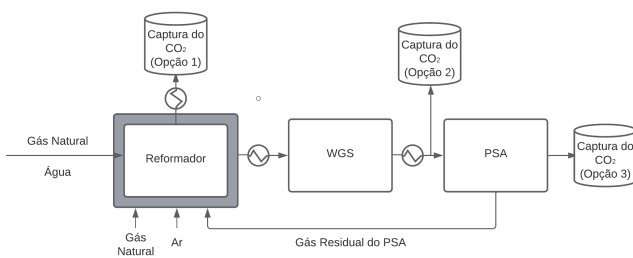
Figura 2. Esquema de uma planta SMR.
