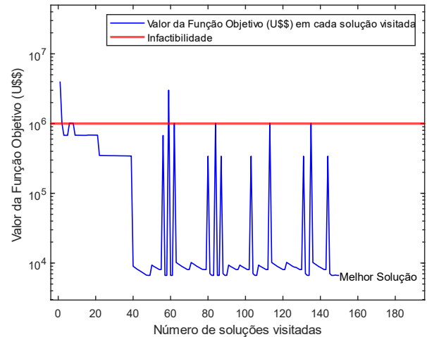
Fig. 4 Valor da função objetivo em todas as soluções visitadas em uma execução do algoritmo ILS proposto.
