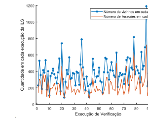
Fig. 8 Quantidade de vizinhos e iterações na execução de verificação.
