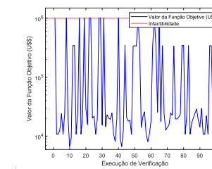
Fig. 7 Valor da função objetivo na execução de verificação.
