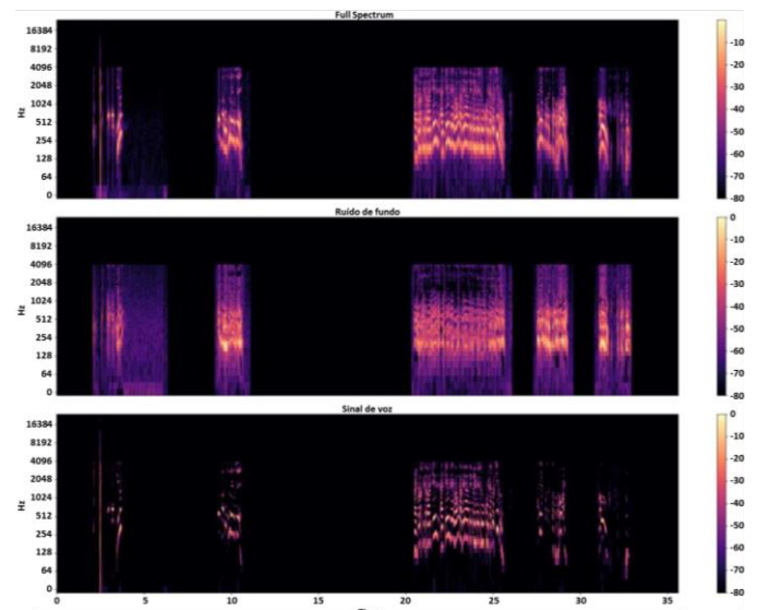
Fig. 8 Análise envolvendo FFT – Canal 1.
