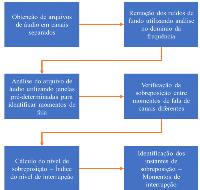
Fig. 7 Fluxograma do módulo de qualidade de chamada.
